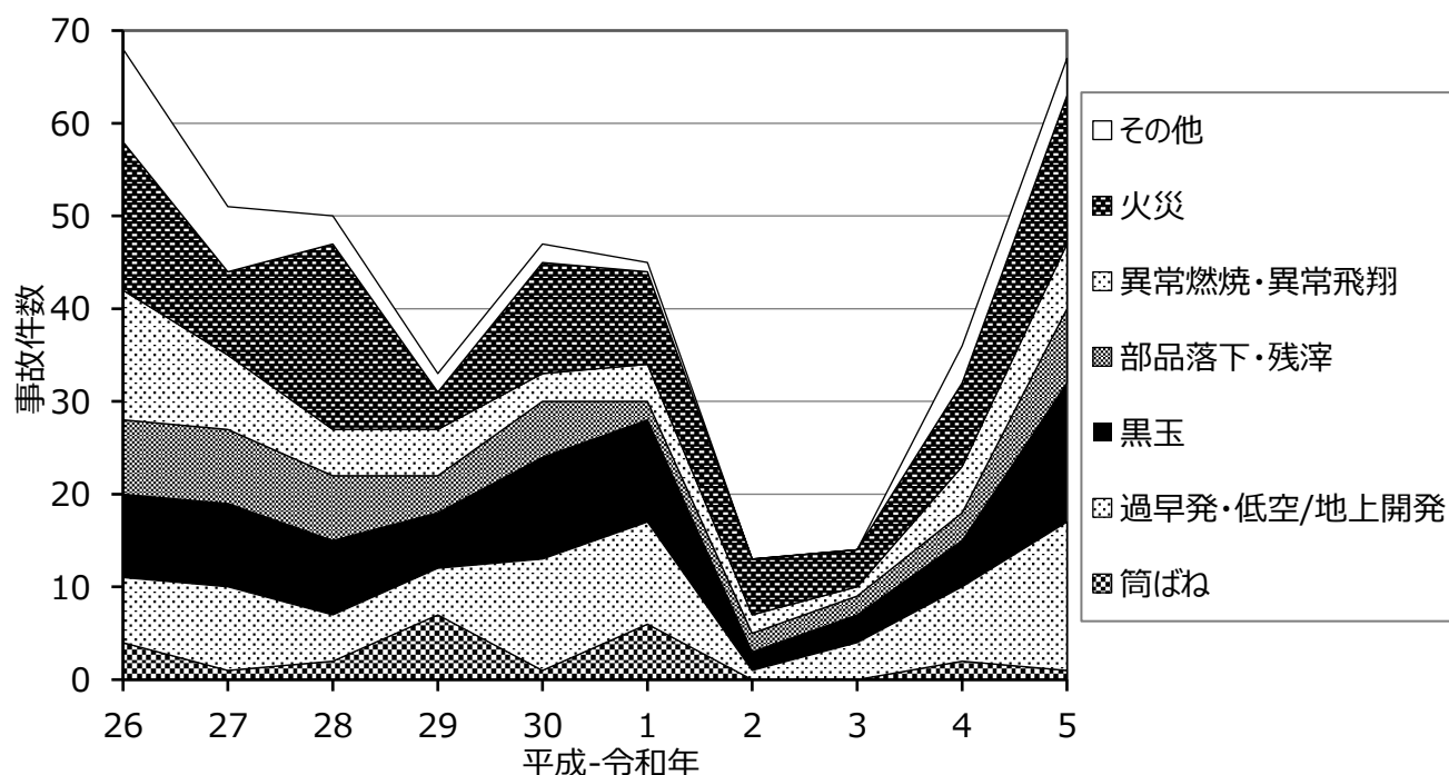
図 5-2 事故現象で分類した過去 10 年の事故件数（煙火消費中）
